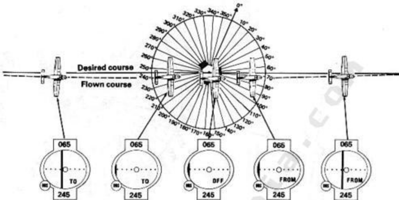
Figure 14. VOR Passage
